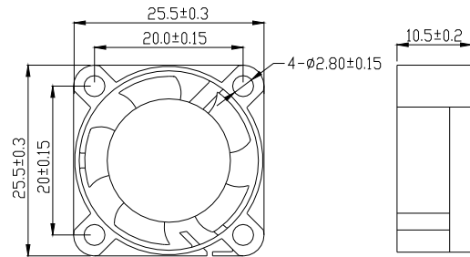
尺寸图 DIMENSIONS DRAWING
